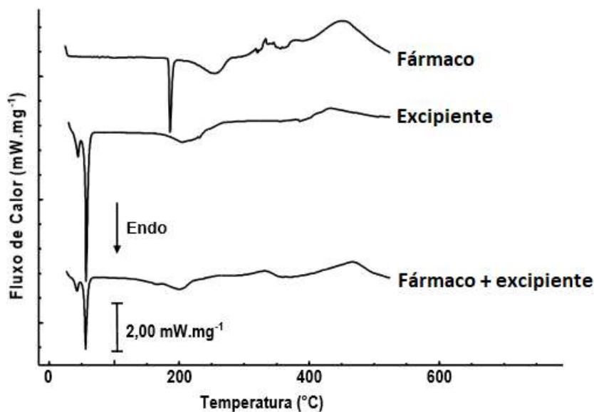
Curva DSC do fármaco, excipiente e da mistura física 1:1 entre estas substâncias obtidas sob atmosfera de N 2 (50 mL/min)
